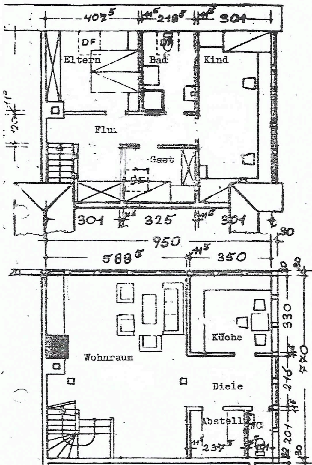
Grundriß Erdgeschoß M. 1: 100
