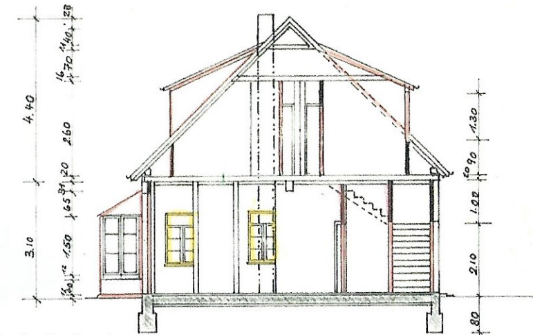
Schnitt A-A
