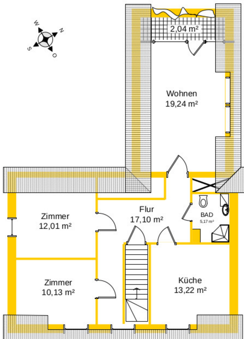
1. OBERGESCHOSS
