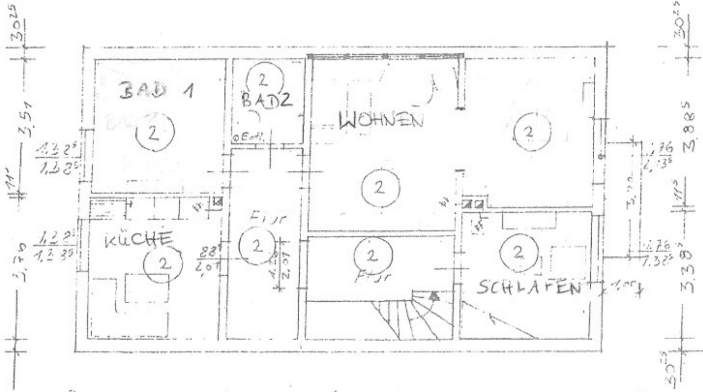
Dachgeschoss - Grundriß
