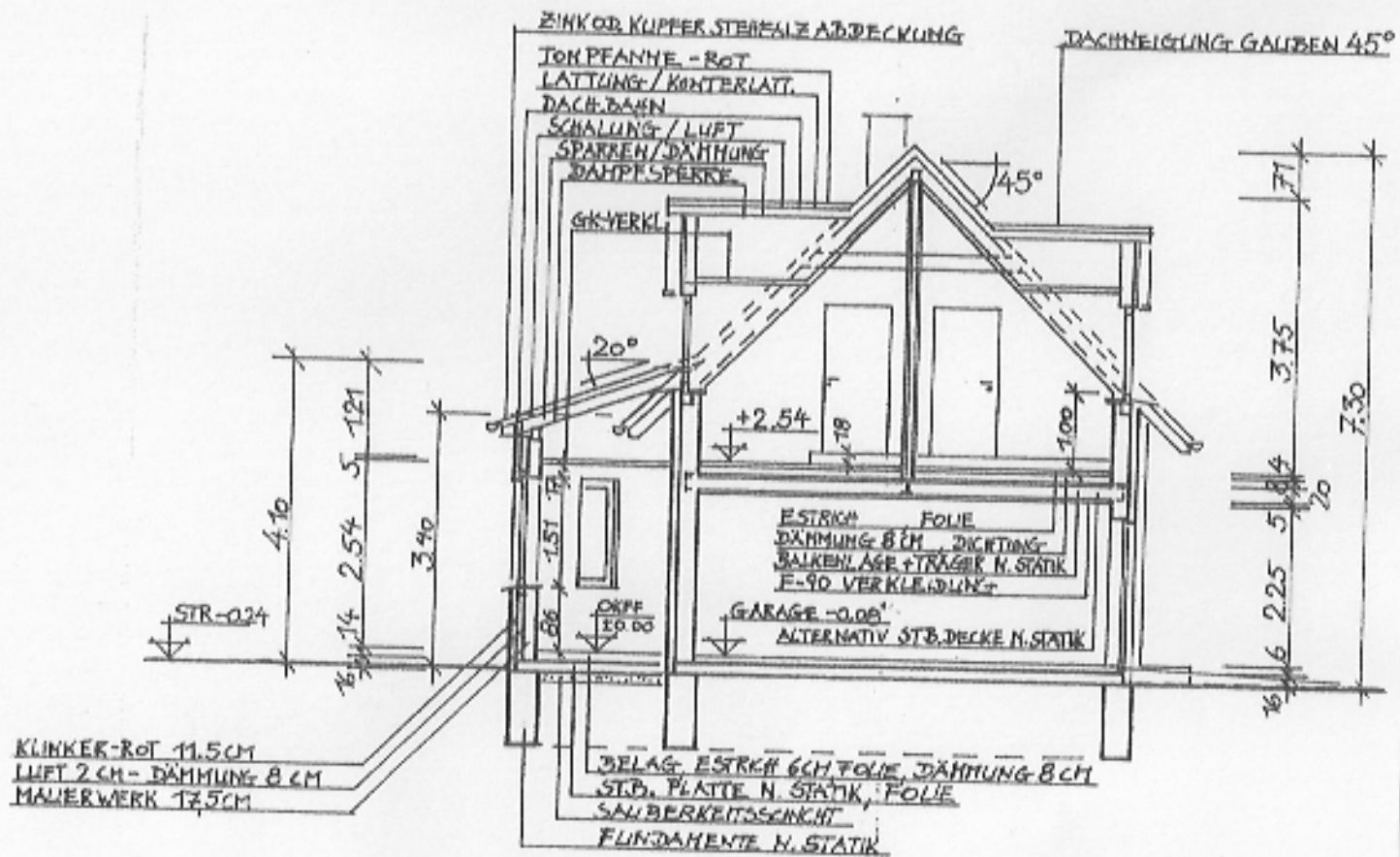
SCHNITT A-A
