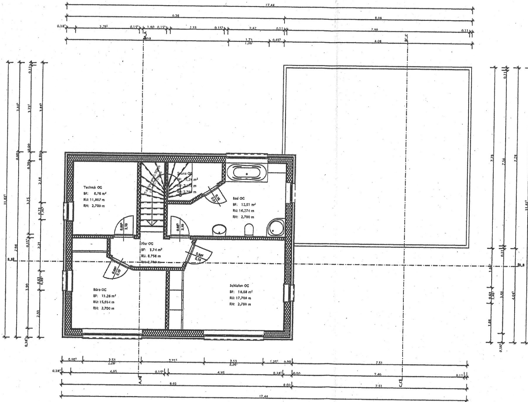
Grundrisse OG M 1:100
